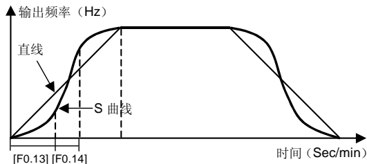
图 6-3 加减速曲线
