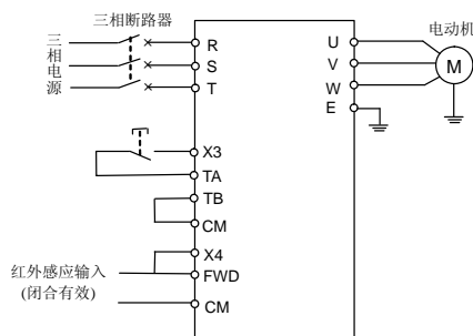
图 9-5 基本接线图
