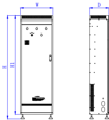
图 2-5 节能柜安装尺寸图
