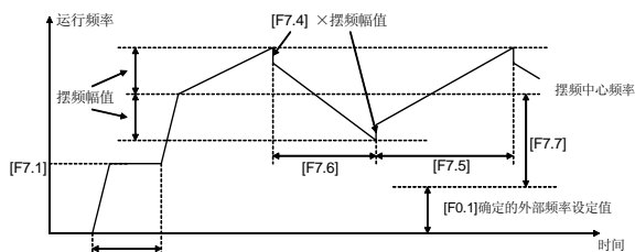
6-27 摆频运行过程
