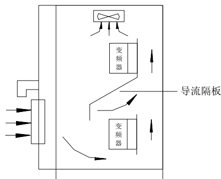
图 2-2 多台变频节能控制柜的安装
