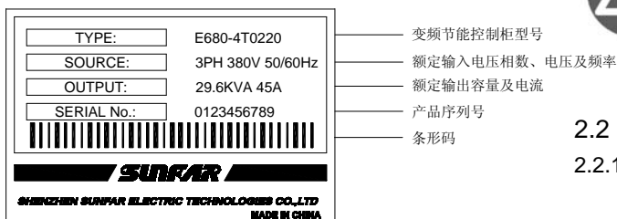
图-1 变频节能控制柜铭牌数据
