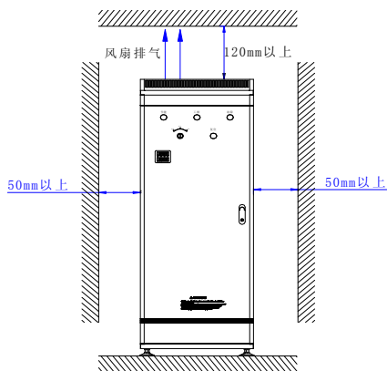
图 2-1 安装的间隔距离
