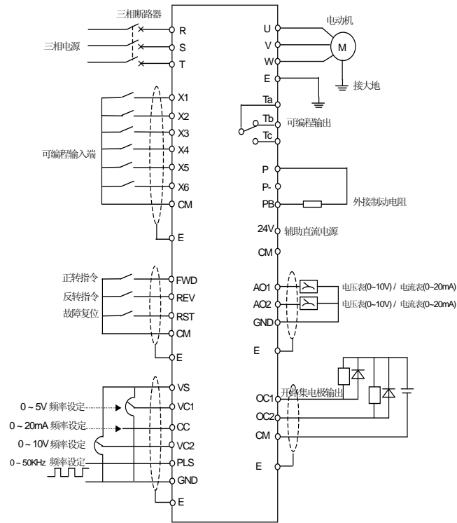
图 3-3 E680 系列变频节能控制柜基本接线
