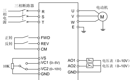
图 9-2 基本接线图
