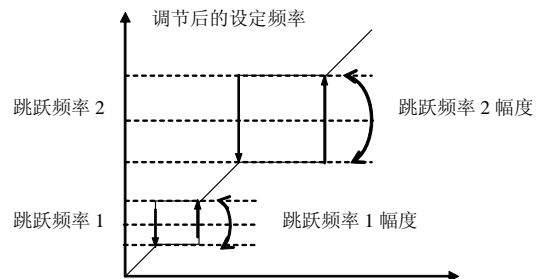
图 6-26 跳跃频率输出
