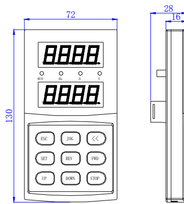
图 2-6 操作面板尺寸图
