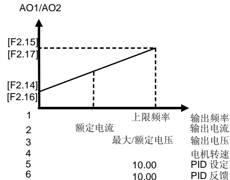
图 6-11 模拟输出端子的模拟输出内容
