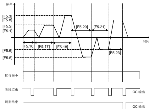
图 6-24a PLC 断点恢复
