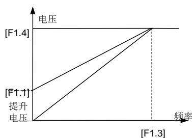
图 6-5 转矩提升
