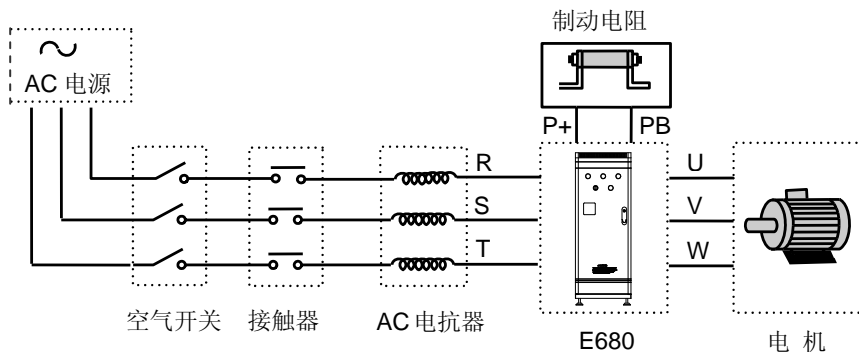
图 3-2 变频节能控制柜的配线
