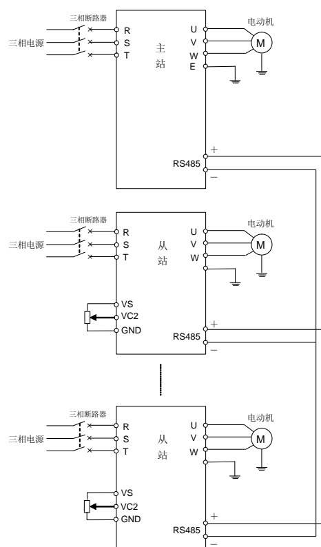
图 9-4 基本接线图
