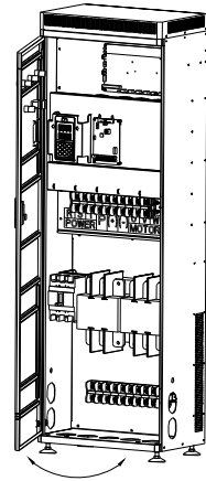
图 2-4 盖板的拆卸和安装
