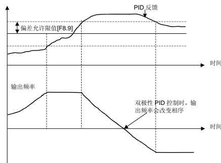
图 6-30 双极性 PID 控制方式
