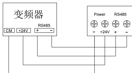
图 C-7 接线方式 2
