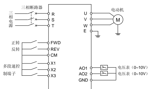
图 9-3 基本接线图
