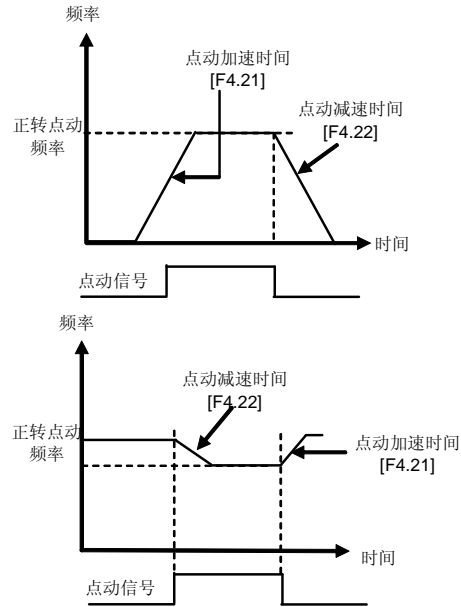
图 6-19 点动运行
